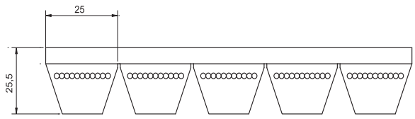
8.20 Pasy klinowe zespolone normalnoprofilowe - profil: 25J5
