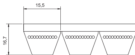
8.14 Pasy klinowe zespolone normalnoprofilowe - profil: 15J3
