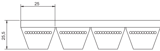
8.19 Pasy klinowe zespolone normalnoprofilowe - profil: 25J4
