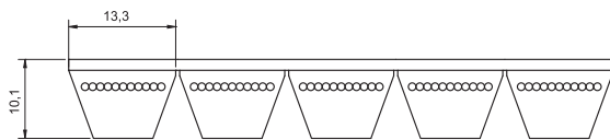
8.10 Pasy klinowe zespolone normalnoprofilowe - profil: 5HA
