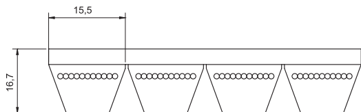
8.15 Pasy klinowe zespolone normalnoprofilowe - profil: 15J4
