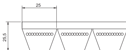
8.18 Pasy klinowe zespolone normalnoprofilowe - profil: 25J3
