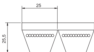
8.17 Pasy klinowe zespolone normalnoprofilowe - profil: 25J2
