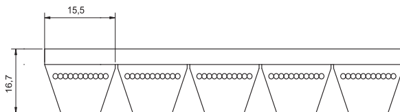
8.16 Pasy klinowe zespolone normalnoprofilowe - profil: 15J5
