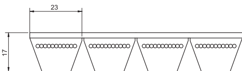
8.9 Pasy klinowe zespolone normalnoprofilowe - profil: 4HC
