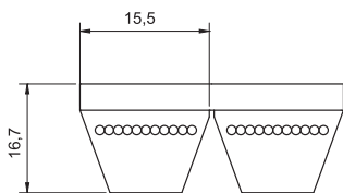
8.13 Pasy klinowe zespolone normalnoprofilowe - profil: 15J2
