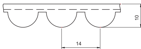
13.13 Pasy zębate - profil: 14M
