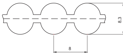
13.15 Pasy zębate - profil: D8M
