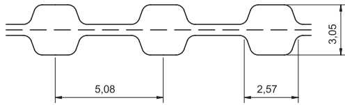
13.7 Pasy zębate - profil: DXL
