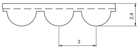
13.10 Pasy zębate - profil: 3M
