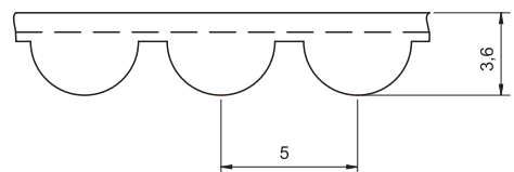
13.11 Pasy zębate - profil: 5M
