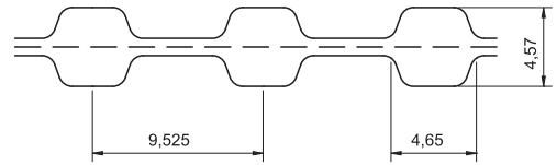
13.8 Pasy zębate - profil: DL
