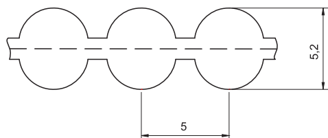
13.14 Pasy zębate - profil: D5M
