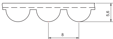
13.12 Pasy zębate - profil: 8M
